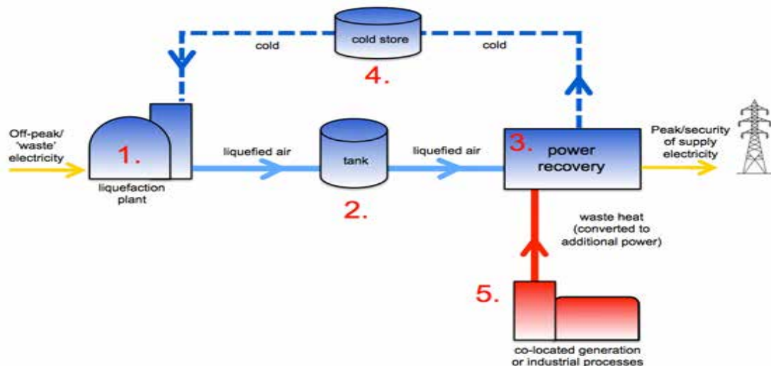
Figur 4.9. Förenklad bild av kryogeniska processen [9].
